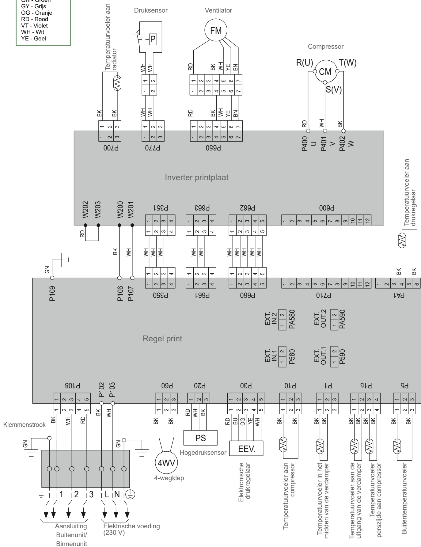
fig. 44 - Elektrische bekabeling van de buitenunit model 10
