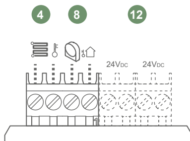
fig. 41 - Voeleraansluitingen
