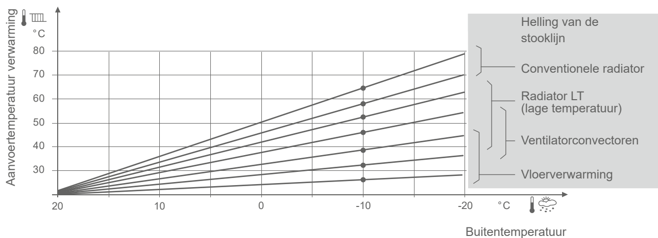
fig. 42 - Helling van de stooklijn
